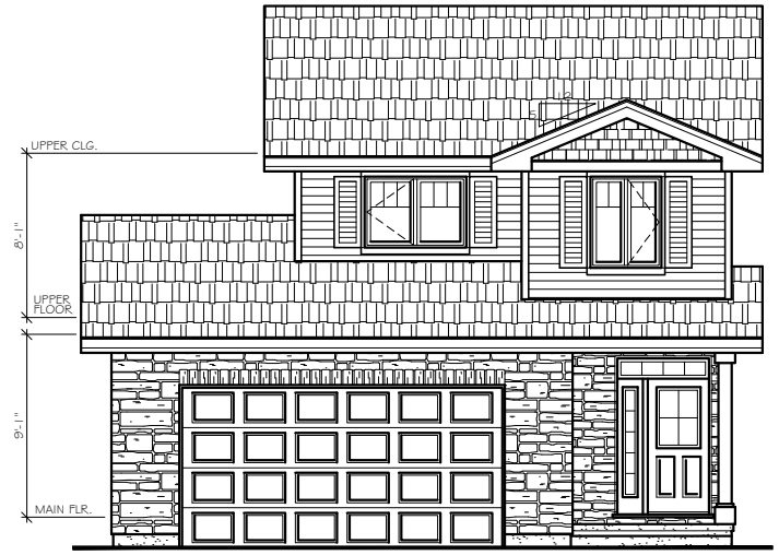
OPTIONAL ELEVATION
